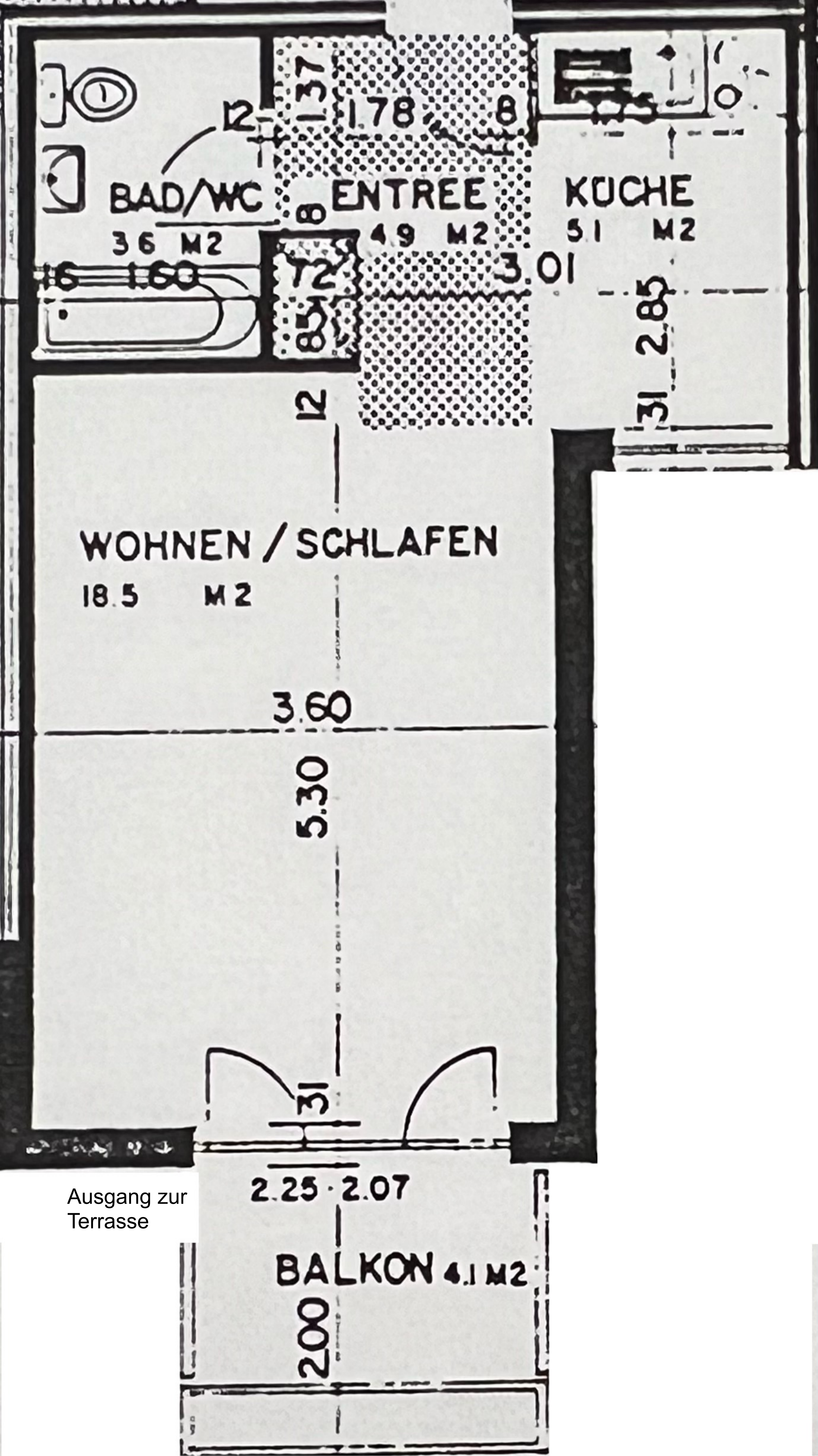
Grundrissplan 1.5-Zi-Wohnung Haus A, Hochparterre, 32m 2 + 15m 2 Terrasse
